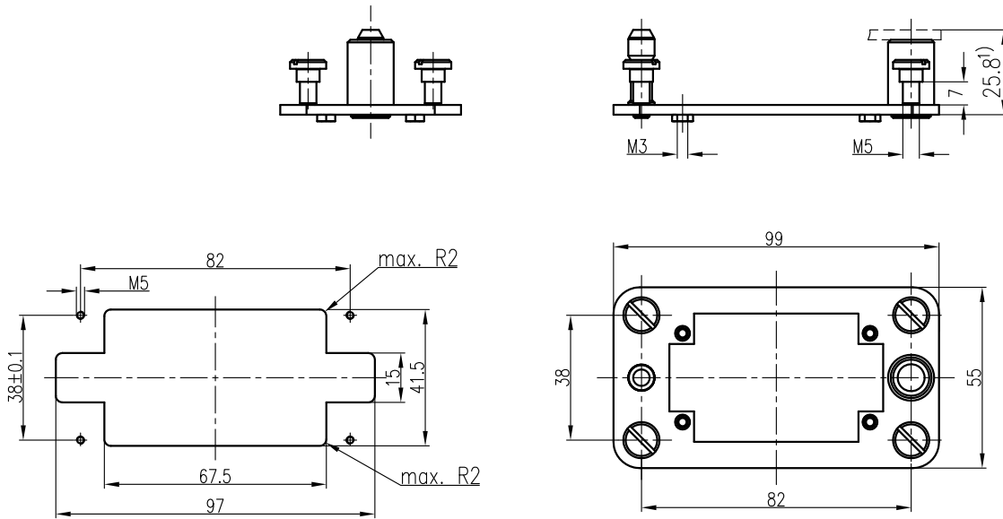
安装开孔图 Panel cut out
