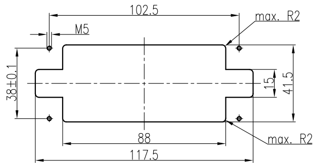
安装开孔图 Panel cut out
