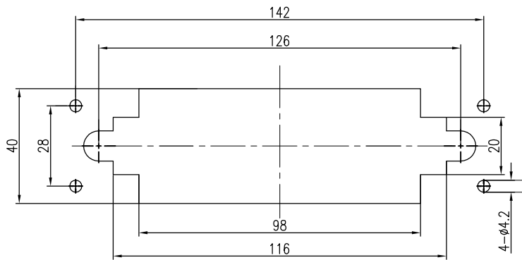
开孔尺寸图
